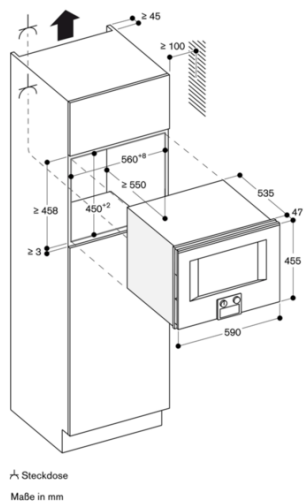
Seitenansicht BS 454/455, BM 454/455 über BO
